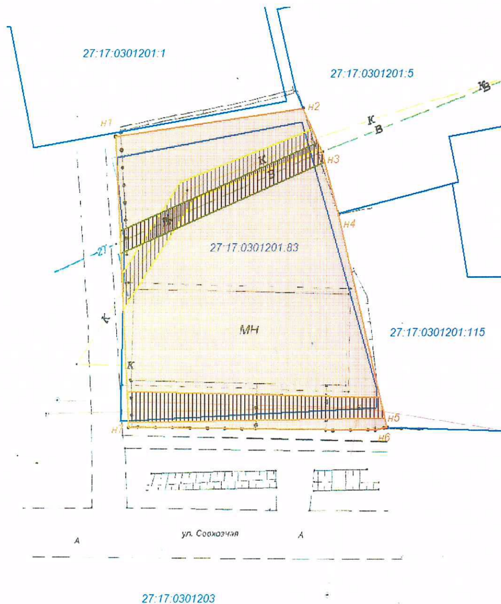
Чертеж проекта межевания территории Масштаб 1:500
